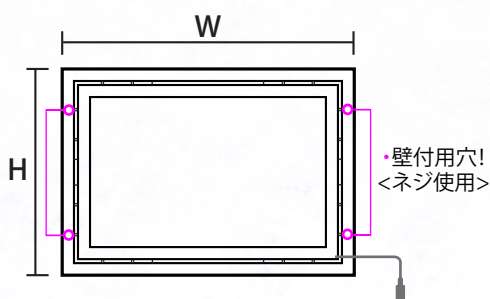
背面図
